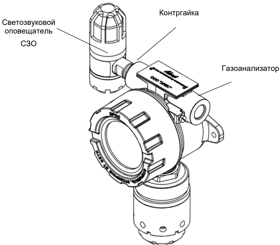
Рисунок 25 – Внешний вид газоанализатора со светозвуковым оповещателем C30
