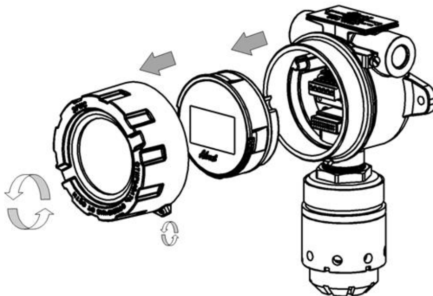
Рисунок 15 – Схема разбора Advant
